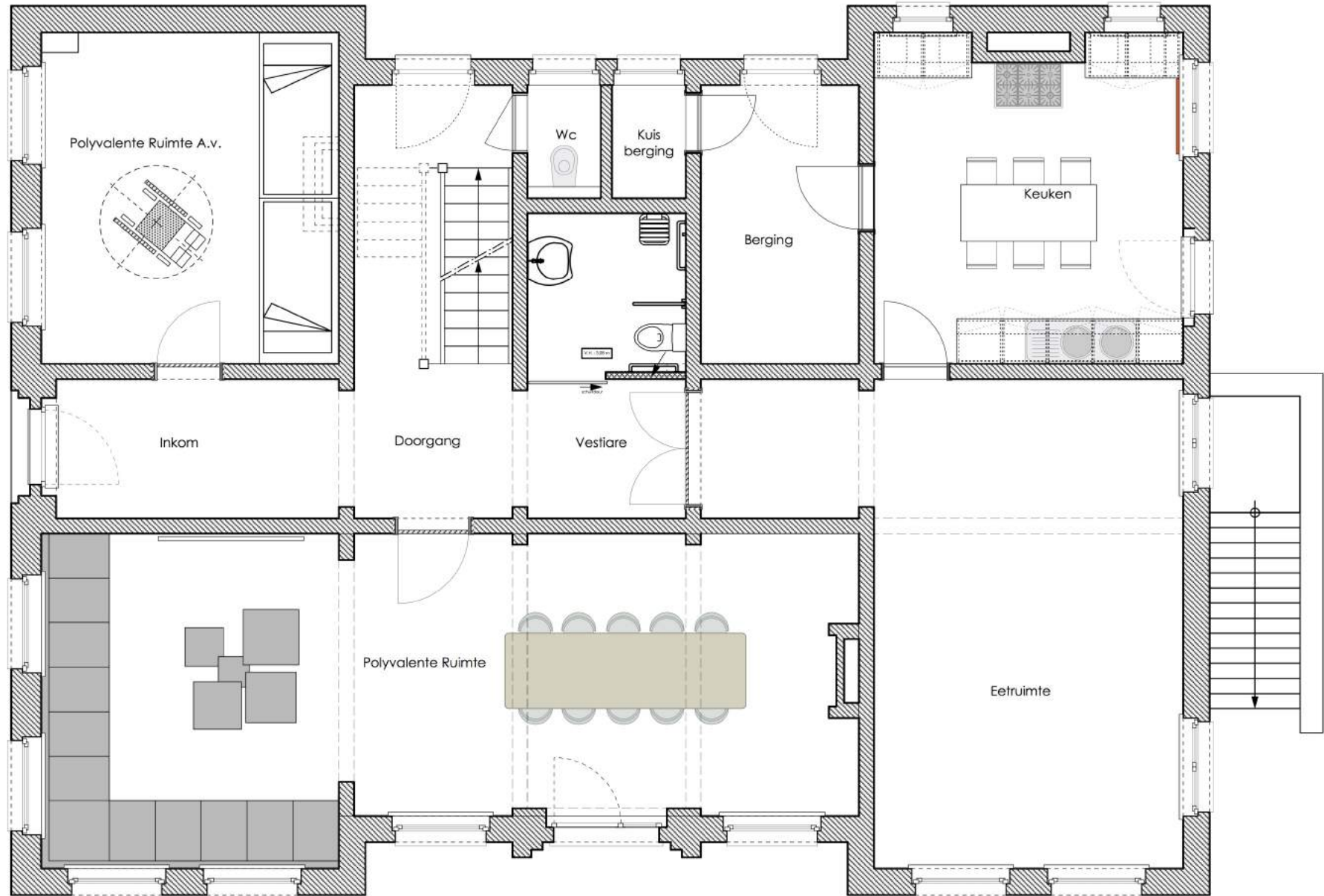
GRONDPLAN
