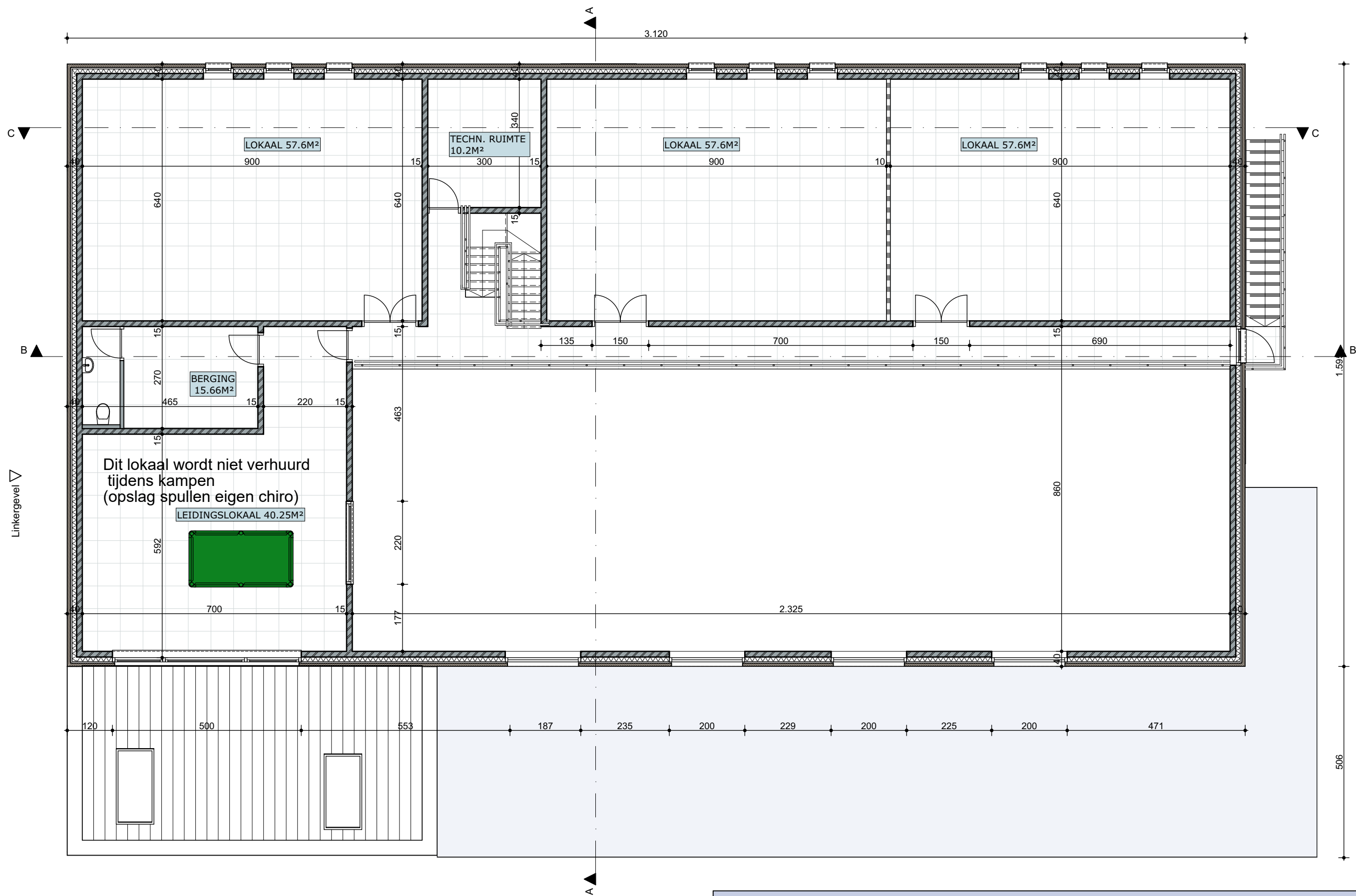
Verdieping+1 Chiro Betekom schaal 1-100
